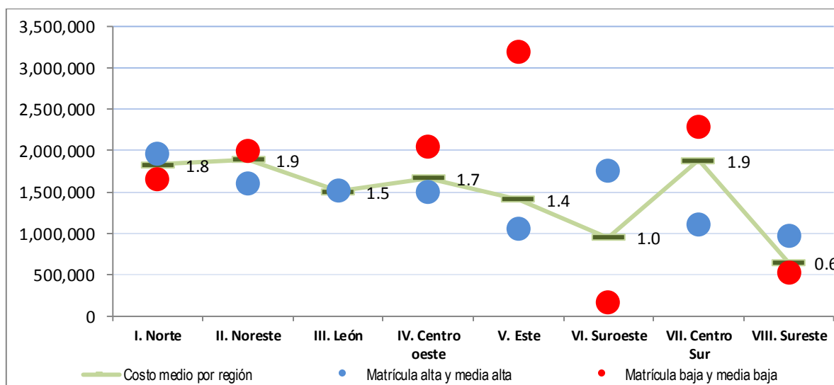
Gráfica 17. Obra. Costos medios por región y tamaño de matrícula
