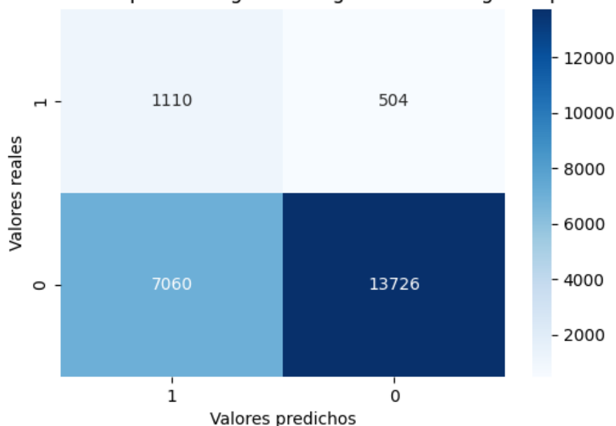
Matriz de confusión para la Regresión Logística en la segunda partición
