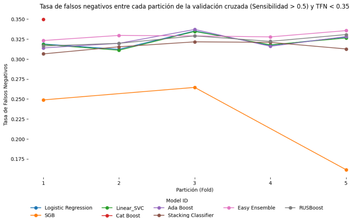
Gráfico III.1 Tasa de falsos negativos entre cada partición de la validación cruzada (sensibilidad > 0.5 y TFN < 0.35)
