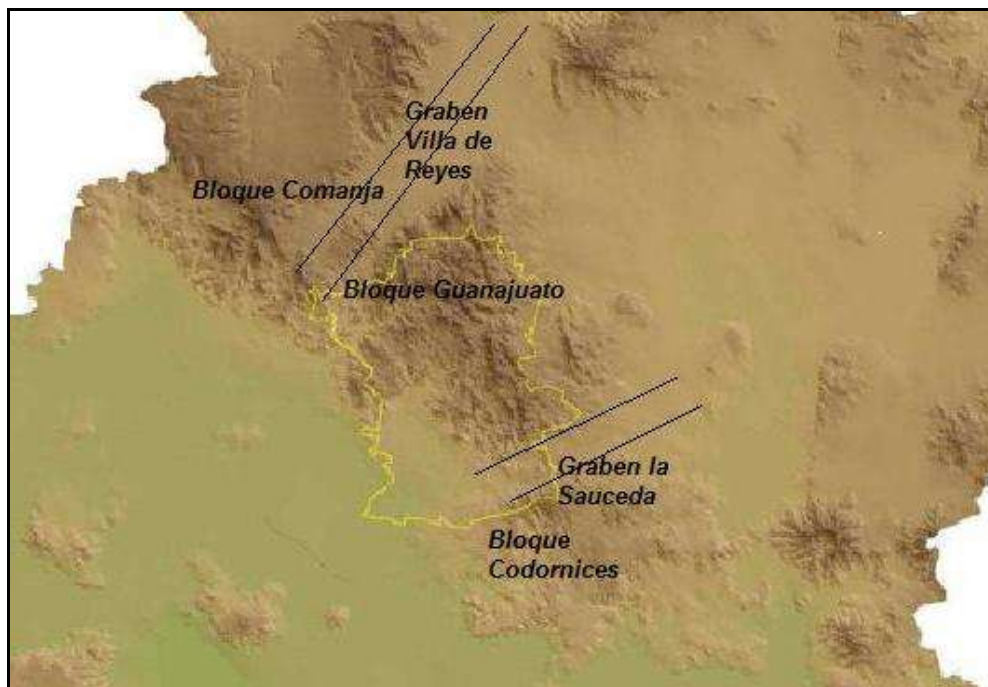
Figura 1. Bloques tectónicos del Municipio de Guanajuato
