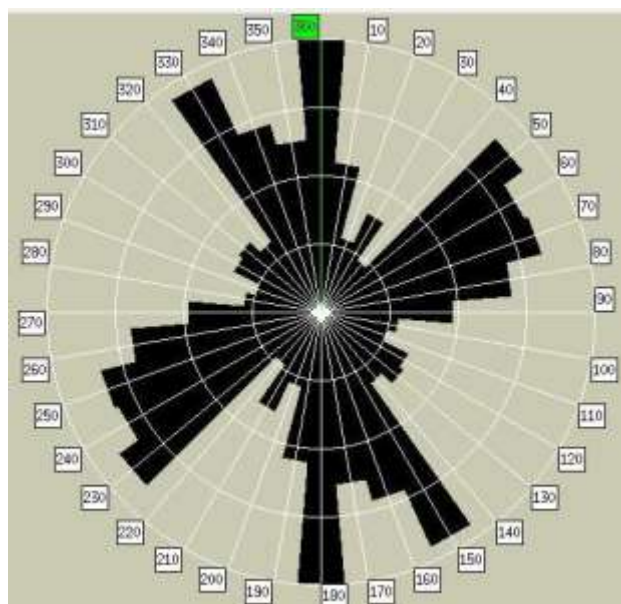
Figura 2. Rosa de alineamientos del fracturamiento y grietas
