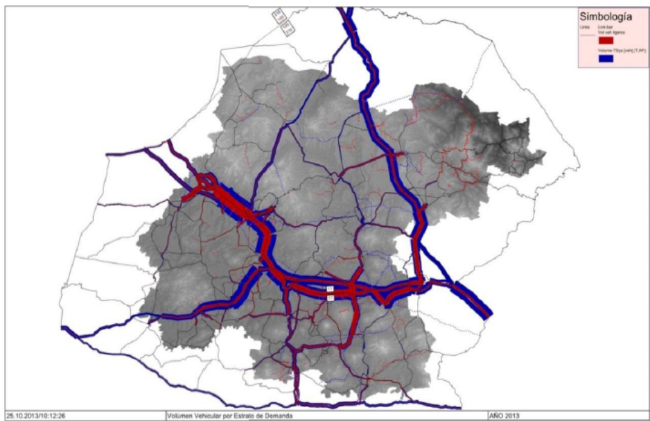
Mapa III.50. Estatal. Tránsito asignado a la red carretera, 2013
