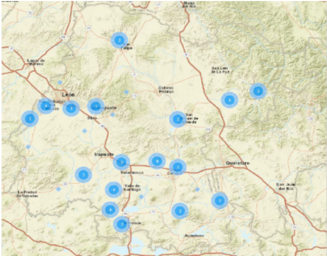
Mapa III.63. Estatal. Puntos de accidentes en carreteras estatales, 2017
