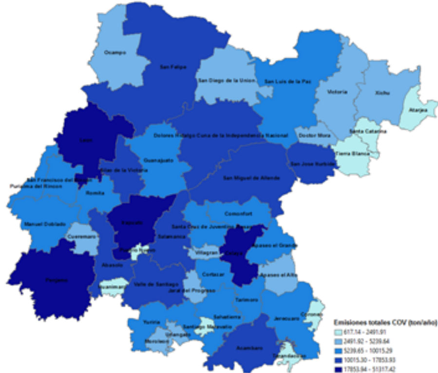
Mapa III.21. Estatal. Distribución geográfica de las emisiones de COV en el estado de Guanajuato, 2013
