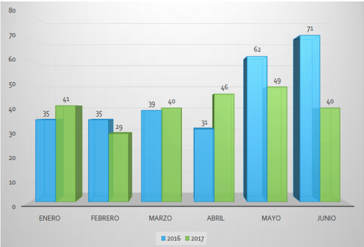
Gráfica III.92. Estatal. Accidentes en carreteras federales, 2017
