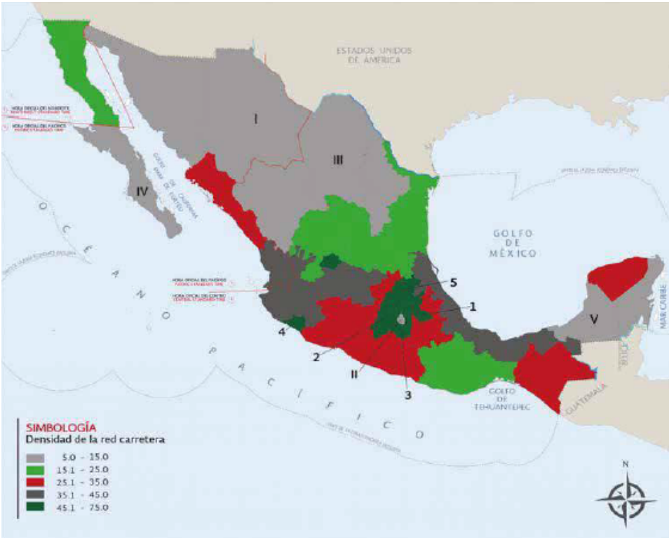
Mapa III.46. Nacional. Densidad de longitud de red carretera por entidad federativa, 2015
