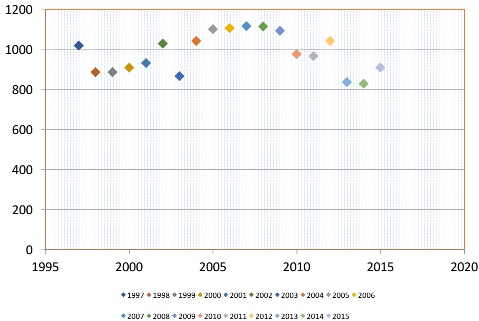
Gráfica III.88. Estatal. Accidentes de tránsito terrestre por colisión con peatón en zonas urbanas y suburbanas, 1997-2015
