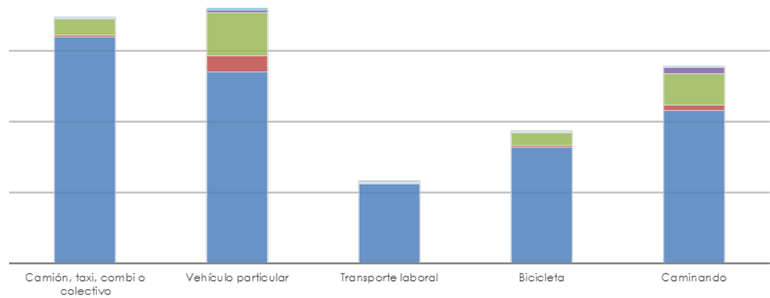
Gráfica III.82. Estatal. Modo de transporte de la población ocupada y por actividad, 2015
