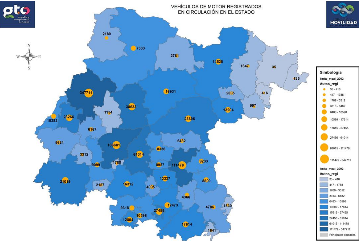
Mapa III.66. Estatal. Automóviles registrados en el estado de Guanajuato, 2016
