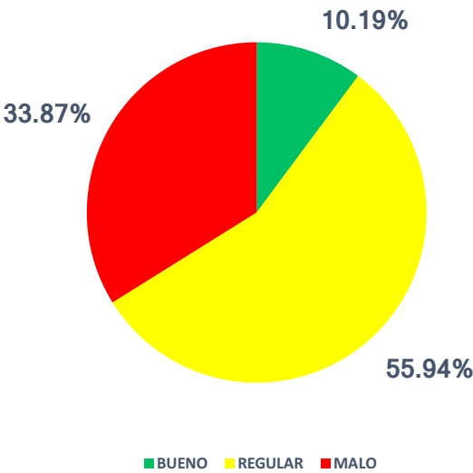
Gráfica III.62. Estatal. Estado de la superficie de rodamiento de las carreteras de jurisdicción federal, 2016
