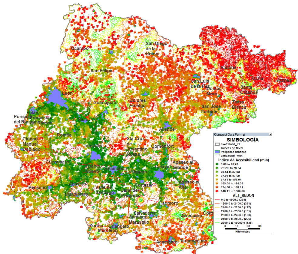
Mapa III.47. Estatal. Accesibilidad de la red carretera, 2016
