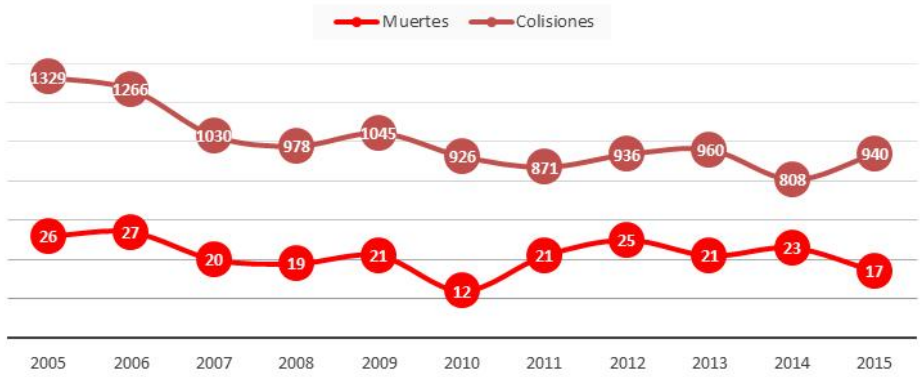
Gráfica III.89. Estatal. Número de accidentes con ciclistas, 2005-2015
