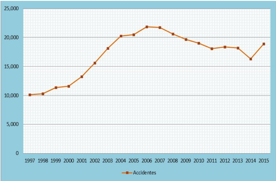
Gráfica III.95. Estatal. Historial de accidentes en el estado, 1997-2015
