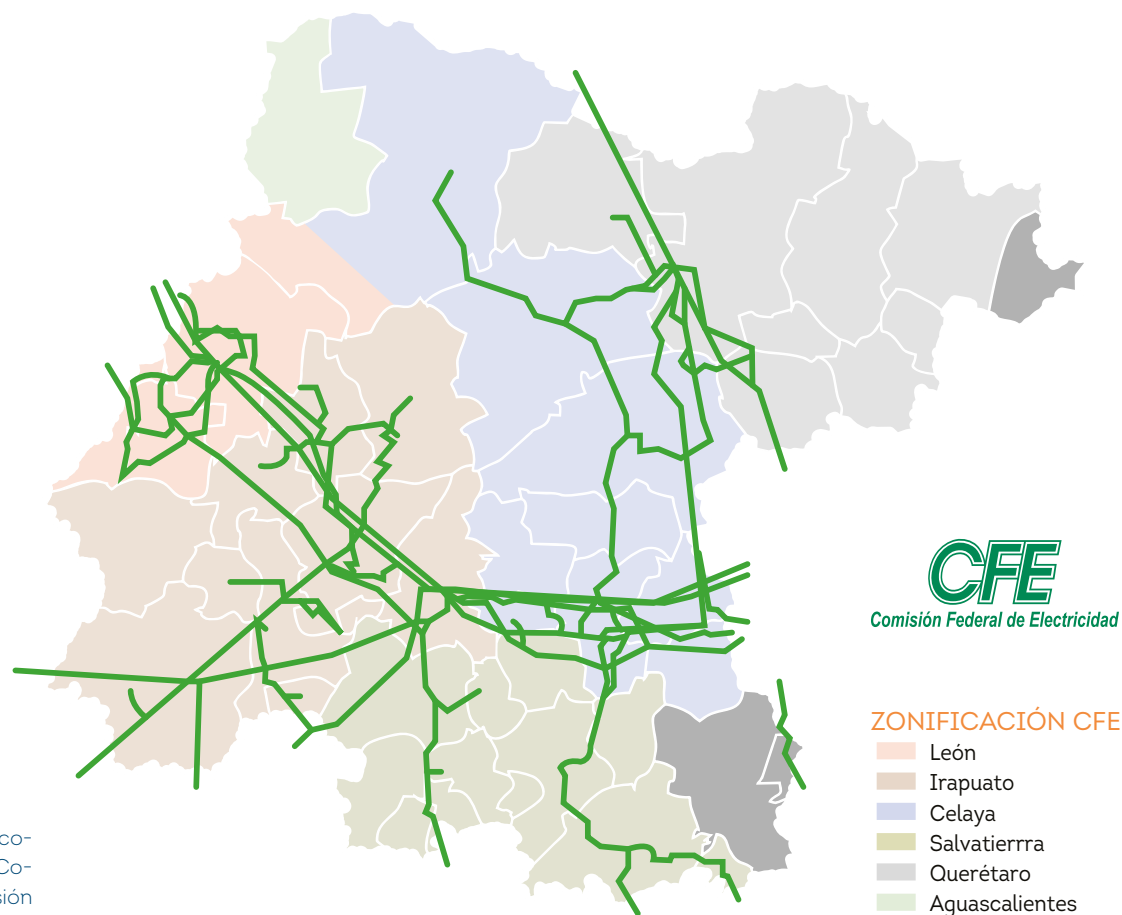
Mapa 2. Estatal. Zonificación de líneas eléctricas de alta tensión de la Comisión Federal de Electricidad.
